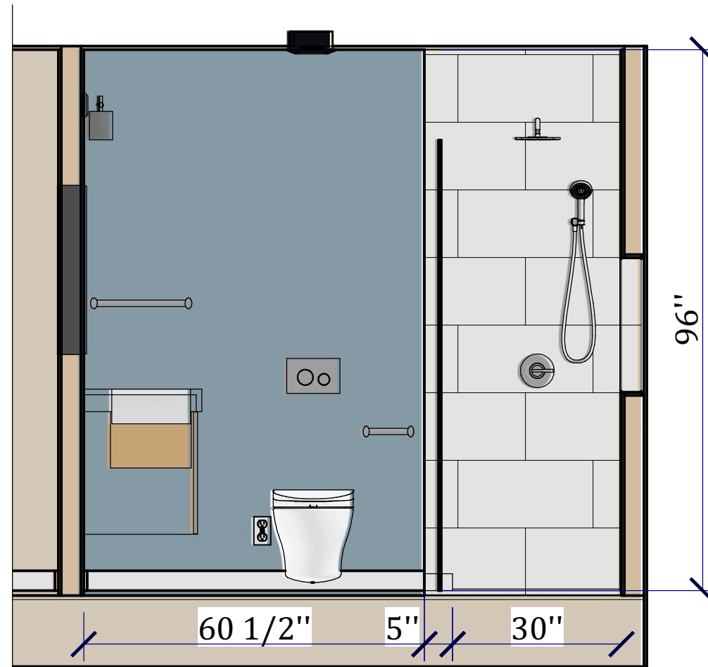
E2 Elevation 1/2"=1'
